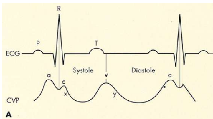
Gambar 12.1: Gelombang CVP
